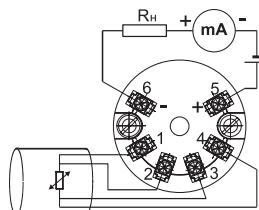
4-х проводная схема подключения ТС
