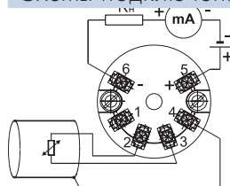
2-х проводная схема подключения ТС
