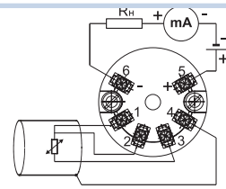
3-х проводная схема подключения ТС
