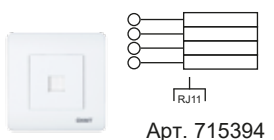
Розетка телефонная 4-проводная
