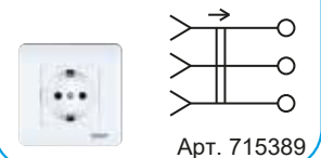
Розетка с заземляющим контактом 16A 250В
