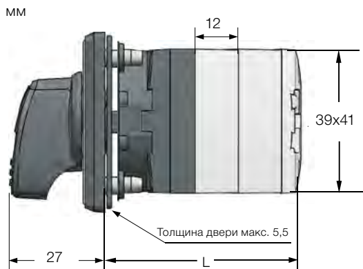
Монтаж привинчиванием, IP66
