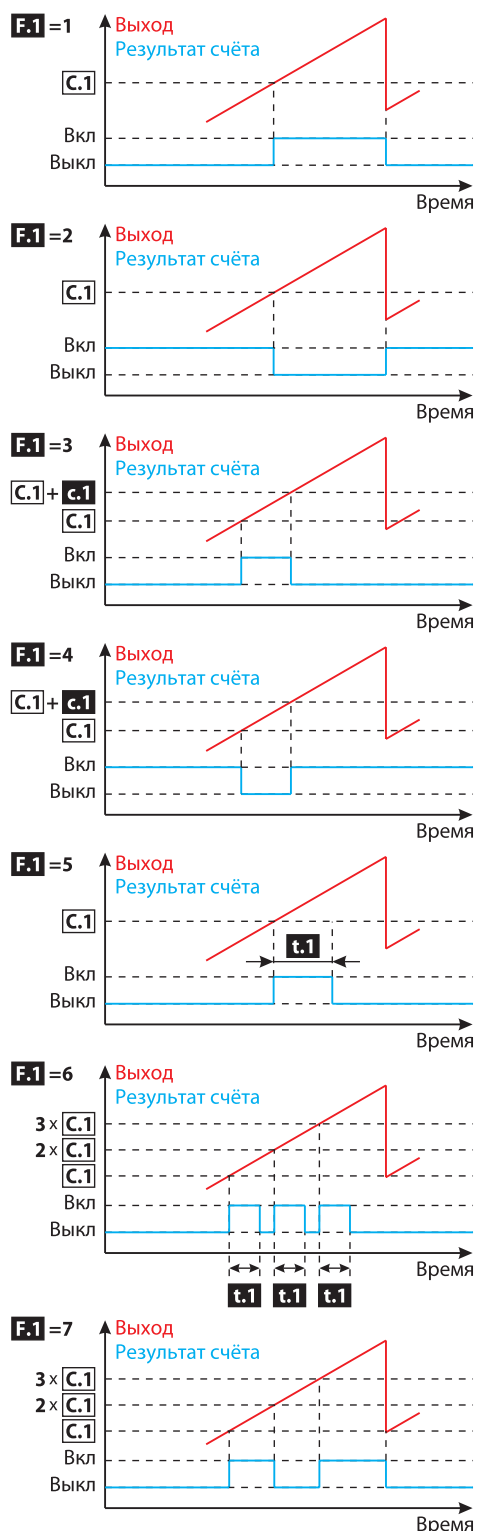
Источники сигнала для компараторов 1, 2
