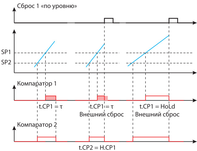
Особенности работы компаратора 2 в случае, когда он подключен к текущему счетчику и его время удержания выбрано равным H.CP1
