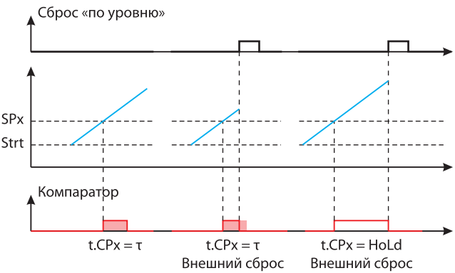
Временная диаграмма работы компараторов
