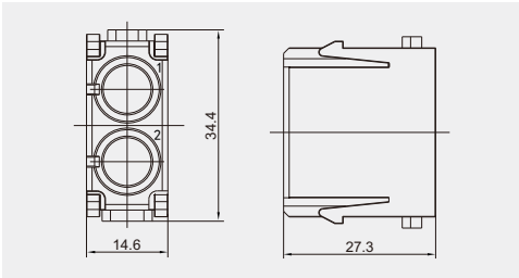
Размеры и расположение отверстия
