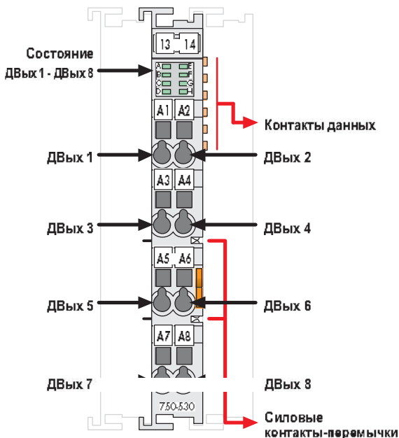
Рис. для серии 750/Технические данные см. на стр. 24/Поставляется без мини-атерных маркеров WSB Маркировку для серий 750/753 см. на стр. 12 - 13/14 - 15
