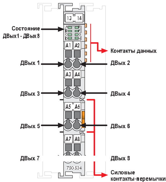
Рис. для серии 750/Технические данные см. на стр. 24/Поставляется без мини-атрипных маркеров WSB Маркировку для серий 750/753 см. на стр. 12 - 13/14 - 16
