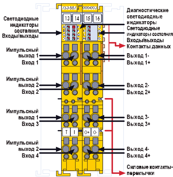
Рис. серии 753/Поставляется без миниатюрных маркеров WSB
