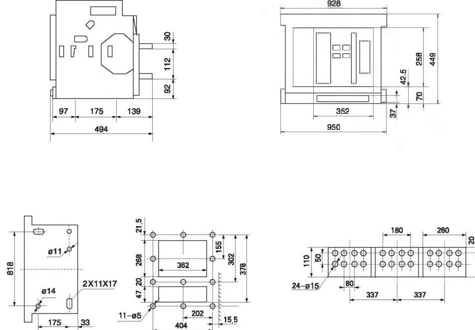
AW45-6300 ВЫДВИЖНОЙ (3-pole)
