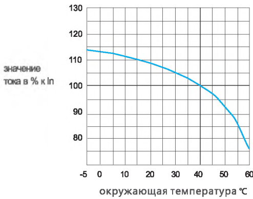
Характеристика температурной зависимости выключателей AM1-250
