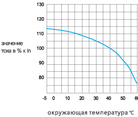
Характеристика температурной зависимости выключателей AM1-1250
