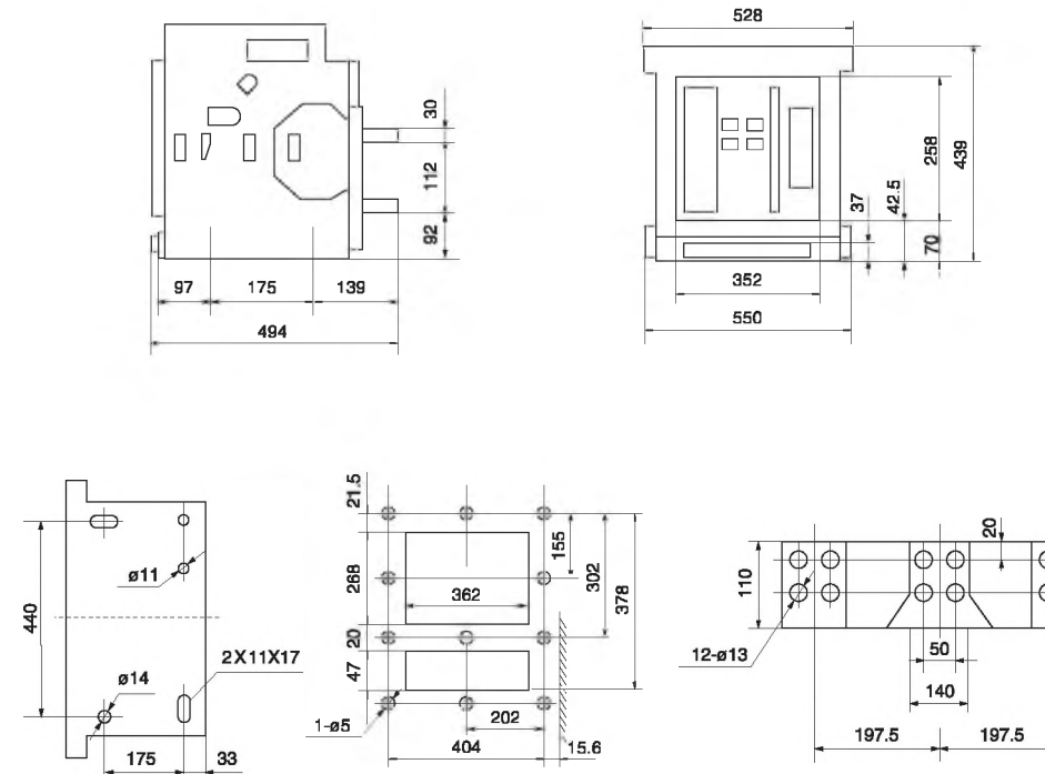
AW45-4000 ВЫДВИЖНОЙ (3-pole)
