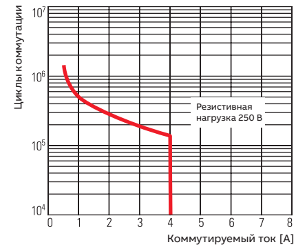
Срок службы контактов
