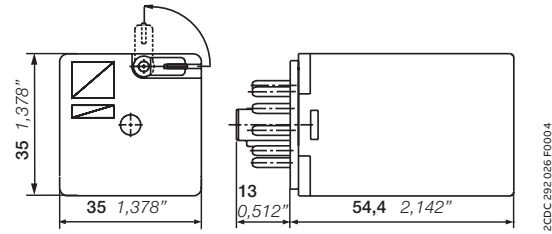
Реле CR-U с 3 переключающими контактами
