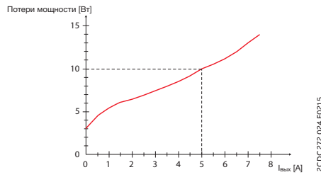
График зависимости средних потерь мощности (тепловыделения) от выходного тока
