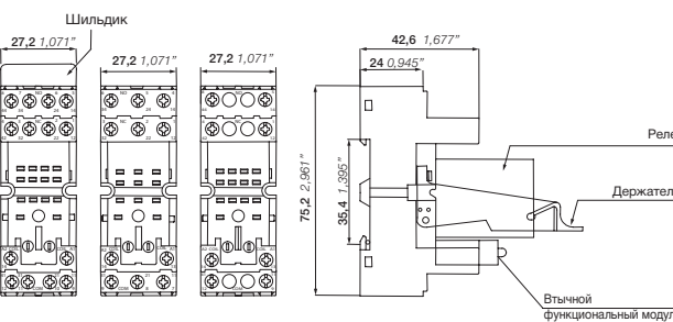
CR-M2SS — CR-M3SS — CR-M4SS с винтовыми клеммами
