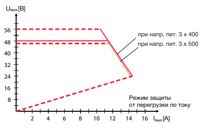
CP-T 48/10.0 Режим прерывания питания (hiccup mode) при перегрузке
