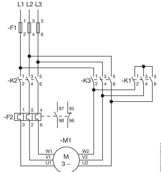
Схема силовой цепи
