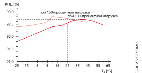
График зависимости среднего КПД от температуры окружающего воздуха
