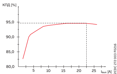
График зависимости среднего КПД от выходного тока
