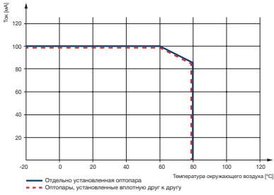
Транзисторный выход CR-S
