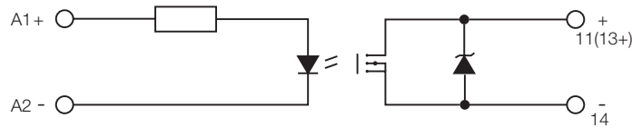
Оптопара CR-S с MOSFET-транзистором
