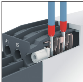
01 Монтаж проводников без инструментов
