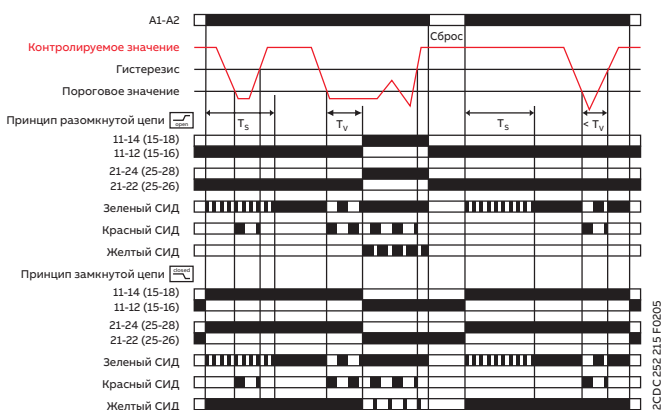
Контроль пониженного тока с функцией памяти
