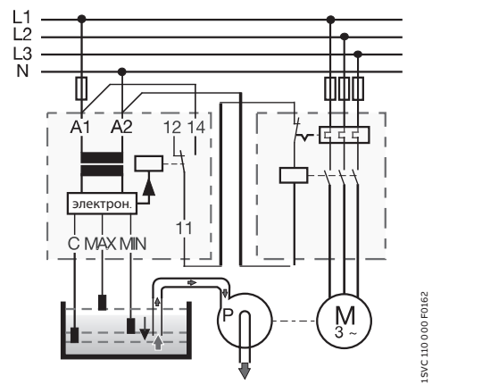
Контроль уровня жидкости — слив: выбрана функция ↓ (DOWN)
