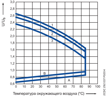
Диапазон рабочего напряжения и температуры катушки постоянного тока
