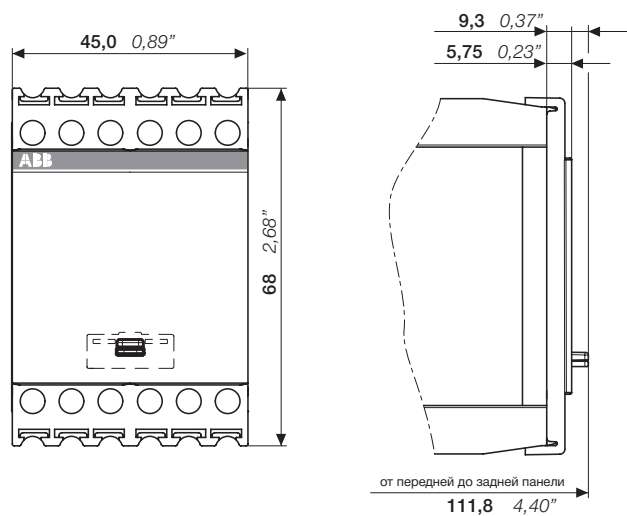
Пломбируемая крышка COV:12
