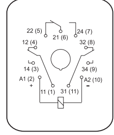
CR-U с 3 переключающими контактами
