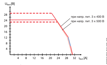
CP-T 24/20.0 Режим снижения напряжения при перегрузке
