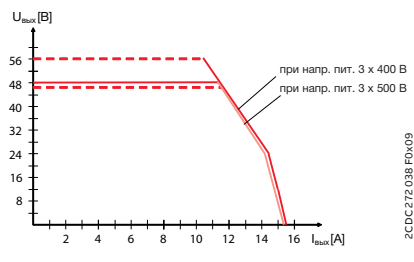
CP-T 48/10.0 Режим снижения напряжения при перегрузке
