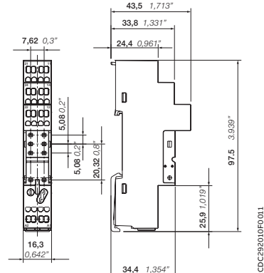
CR-PLS с пружинными клеммами
