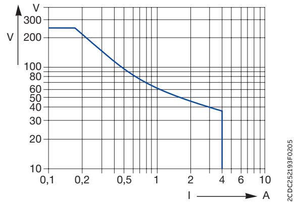
Нагрузка DC (резистивная)
