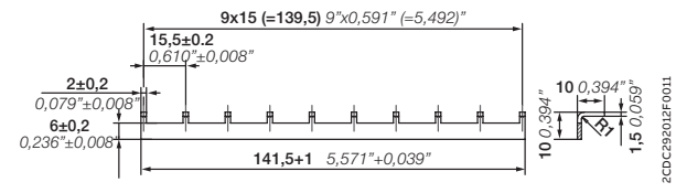
Перемычка CR-PJ
