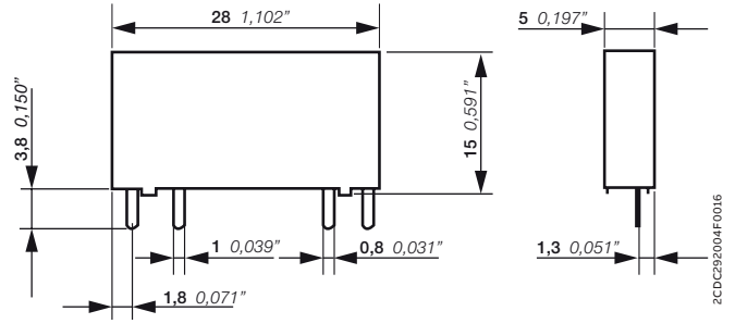
Оптопара CR-S
